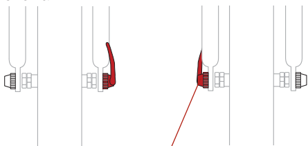
Roue réorientée, avec levier de démontage rapide du côté opposé
